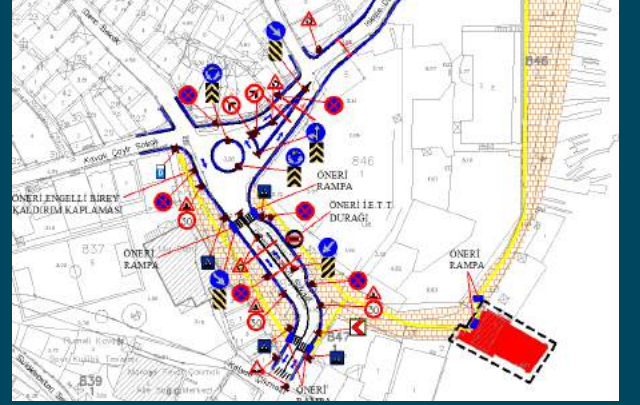
Geometrik Düzenlemeler
